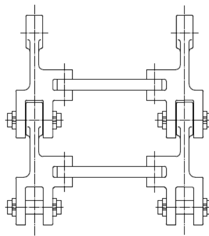
Double Link
